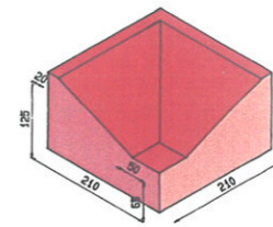
Formanshluß 90° äußere Biegung
