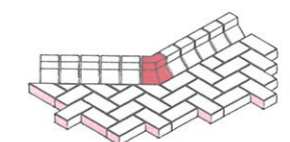
"Buckfast" (hoch) 45° äußere Biegung
