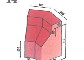
"Buckfast" (hoch) 90° innere Biegung
