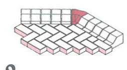
"Buckfast" 45° sich in einem Winkel treffende innere Biegung
