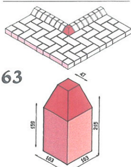
Geneigte Bordkante 90° äußere Biegung
