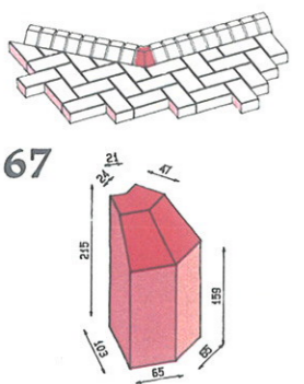
Geneigte Bordkante infultriert 45° innere Rückgang
