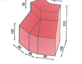
"Buckfast" (hoch) 45° sich in einem Winkel treffende innere Biegung
