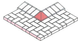
"Nantwich" 90° äußere Biegung
