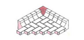
"Buckfast" (hoch) 90° innere Biegung
