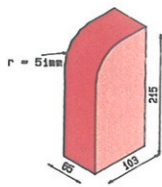
Bullnose 90° äußere Biegung
