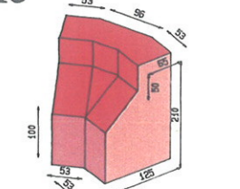
"Buckfast" (hoch) 90° sich in einem Winkel treffende innere Biegung
