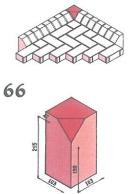
Geneigte Bordkante 90° innere Rückgang
