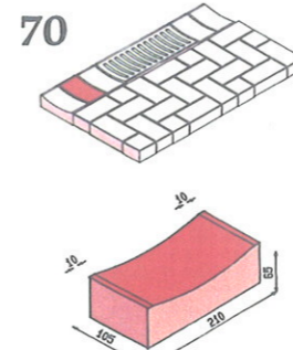
Kanaleinheit inklusive Kanalgitter
