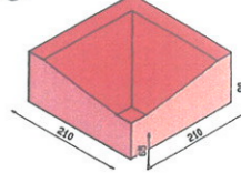
"Carlisle" Bordkante 45° äußere Biegung
