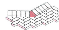
Formanshluß 45° äußere Biegung
