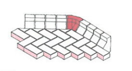
"Buckfast" (hoch) 45° sich in einem Winkel treffende innere Biegung
