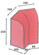
Schräge "Bullnose" Bordkante (Satz v. 4 Einheiten)
