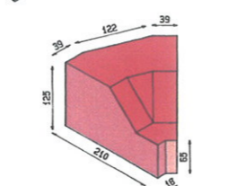
"Buckfast" 45° sich in einem Winkel treffende äußere Biegung
