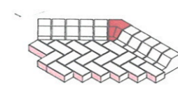
"Buckfast" 45° innere Biegung
