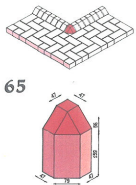
Geneigte Bordkante 90° äußere Rückgang
