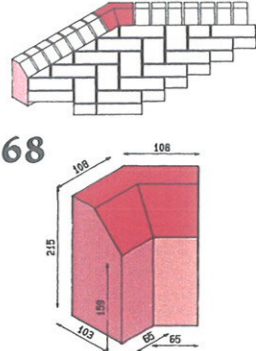
Geneigte Bordkante 45° innere Rückgang
