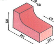
"Abbey" Bordkante 90° äußere Biegung
