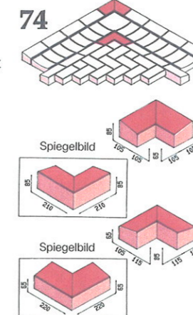
Erweiterte Kanalbiegung 90° (Satz v. 2 Einheiten)
