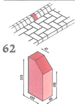
Geneigte Bordkante
