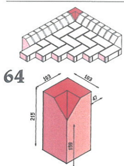
Geneigte Bordkante 90° sich in einem Winkel treffende äußere Biegung
