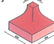
"Abbey" Bordkante 90° innere Biegung
