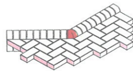
Bullnose 45° äußere Biegung
