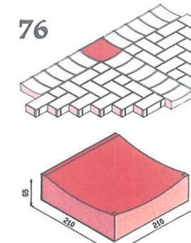
Kanal T-Verbindungseinheit
