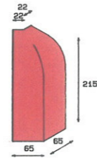
Bullnose 45° innere Biegung
