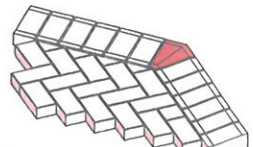
"Carlisle" Bordkante 45° innere Biegung
