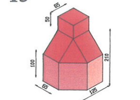
"Buckfast" (hoch) 45° äußere Biegung
