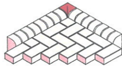
Bullnose 90° innere Biegung
