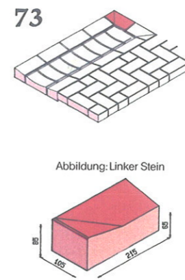
Erweitertes Schlußstück (Satz v. 2 Einheiten)
