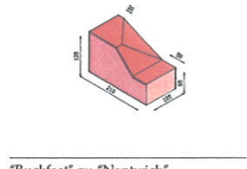
"Buckfast" zu "Nantwich" Übergang Einheit
