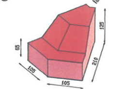
"Buckfast" 45° sich in einem Winkel treffende äußere Biegung
